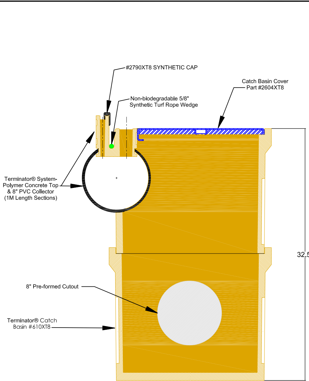
SECTION A-A
